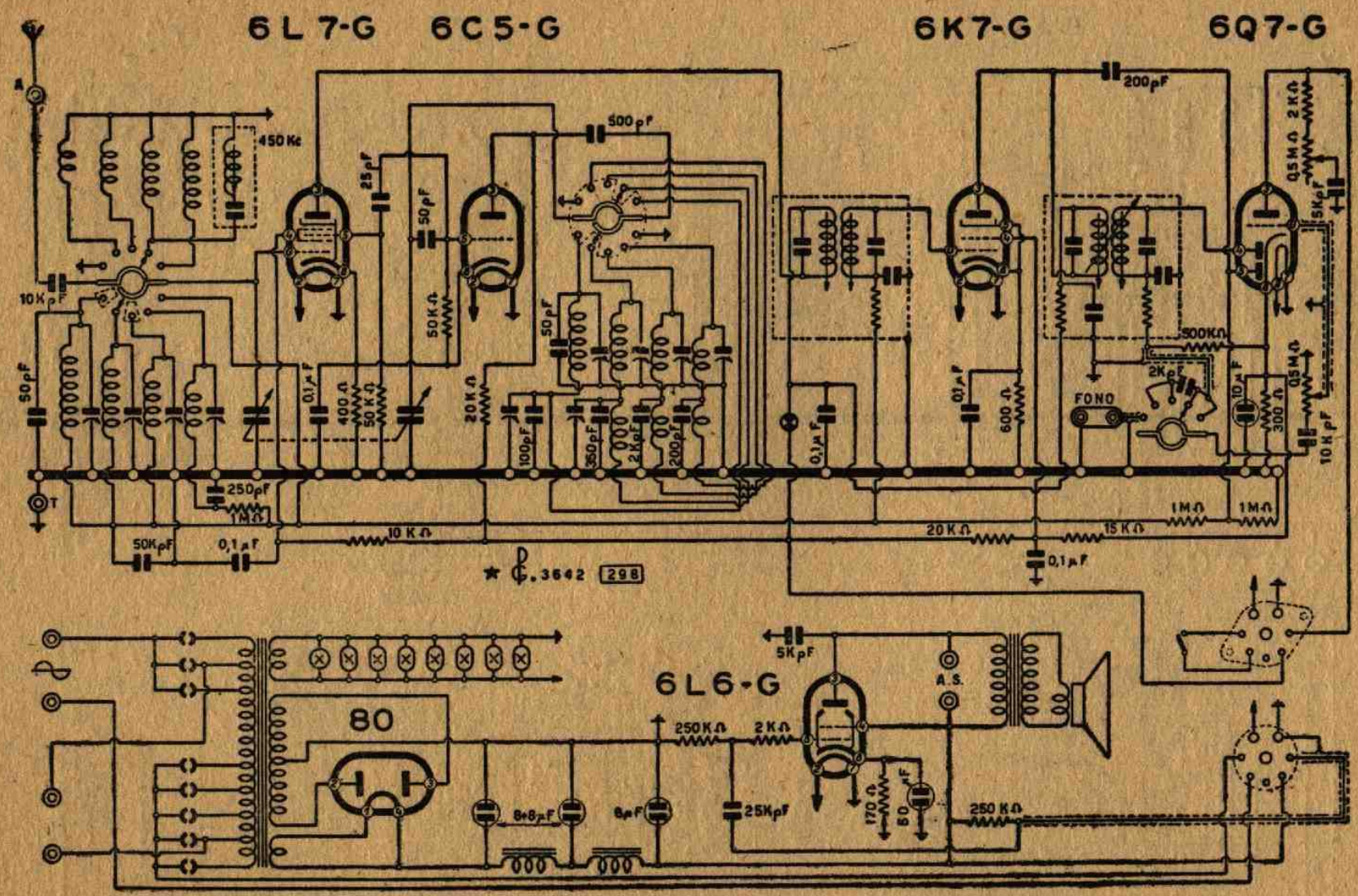
Lo schema elettrico del Super Quadri - Unda 639.
